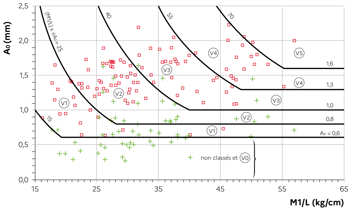
Figure 14: Diagramme de classement des compacteurs vibrants monocylindres
